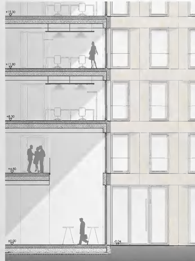
Fassadenanschnitt
