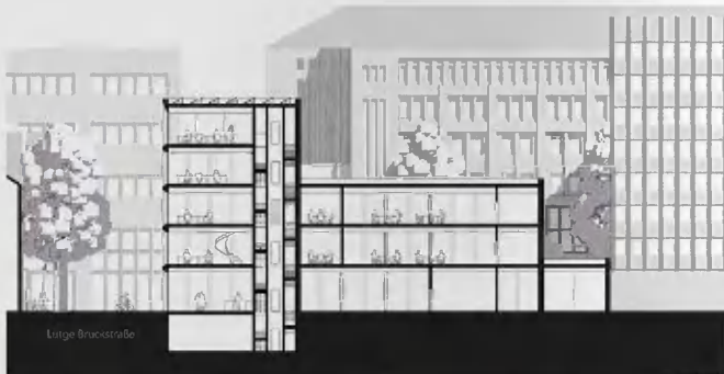
Schnitt EA
