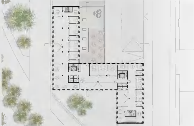
Grundriss 2.06
